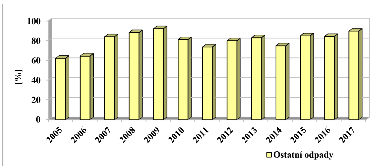
Graf č. 7: Podíl využitých ostatních odpadů letech 2005 – 2017.
