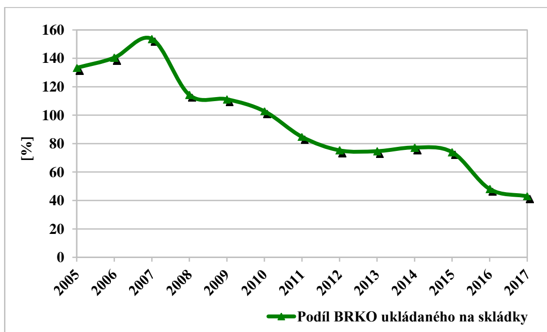
Graf č. 25: Podíl BRKO ukládaného na skládky v letech 2005 – 2017 vzhledem ke srovnávací základně z roku 1995.
