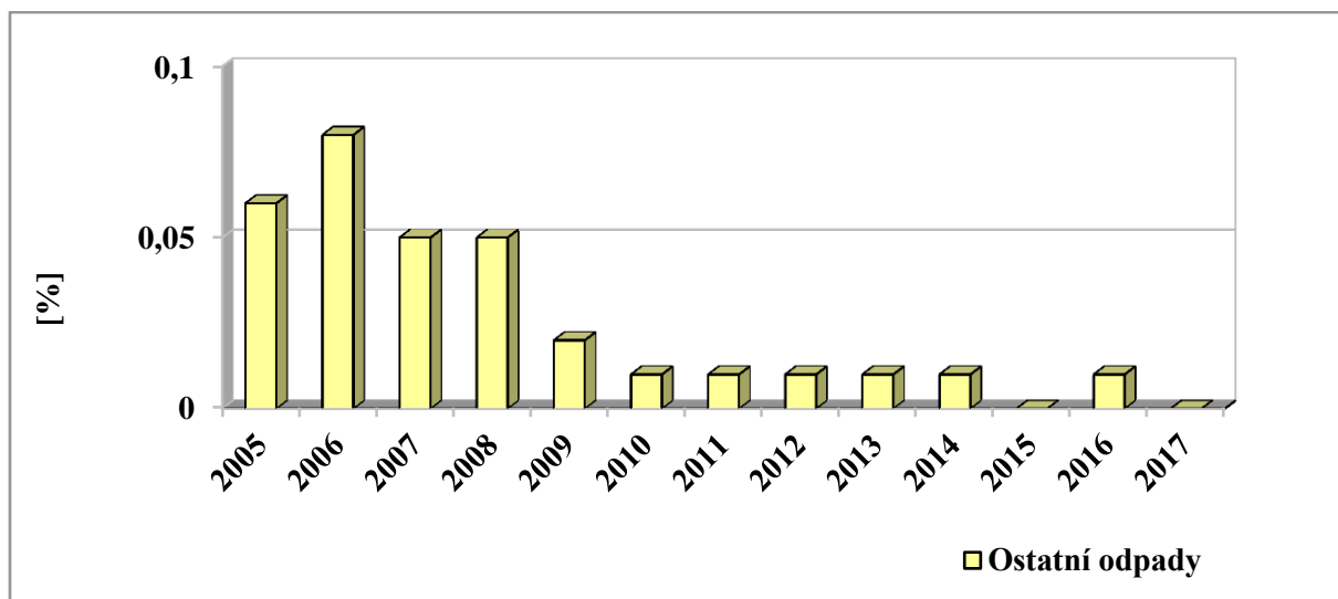
Graf č. 22: Podíl ostatních odpadů odstraněných spalováním v letech 2005 – 2017.
