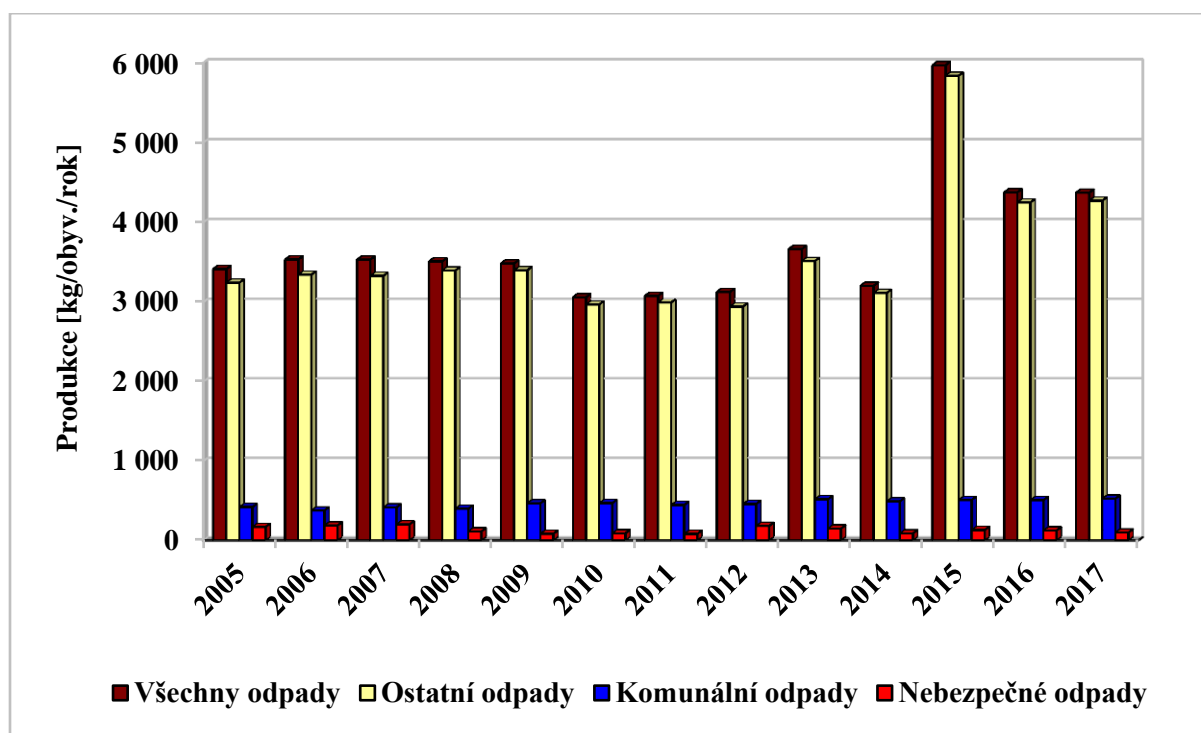
Graf č. 3: Produkce odpadů na obyvatele v letech 2005 – 2017.
