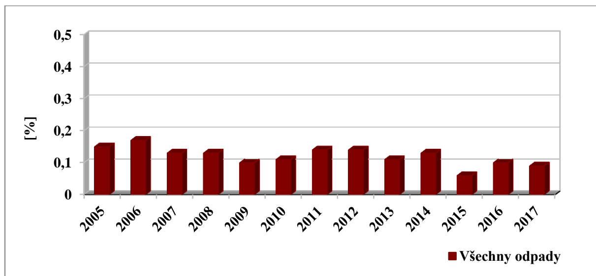
Graf č. 20: Podíl všech odpadů odstraněných spalováním v letech 2005 – 2017.
