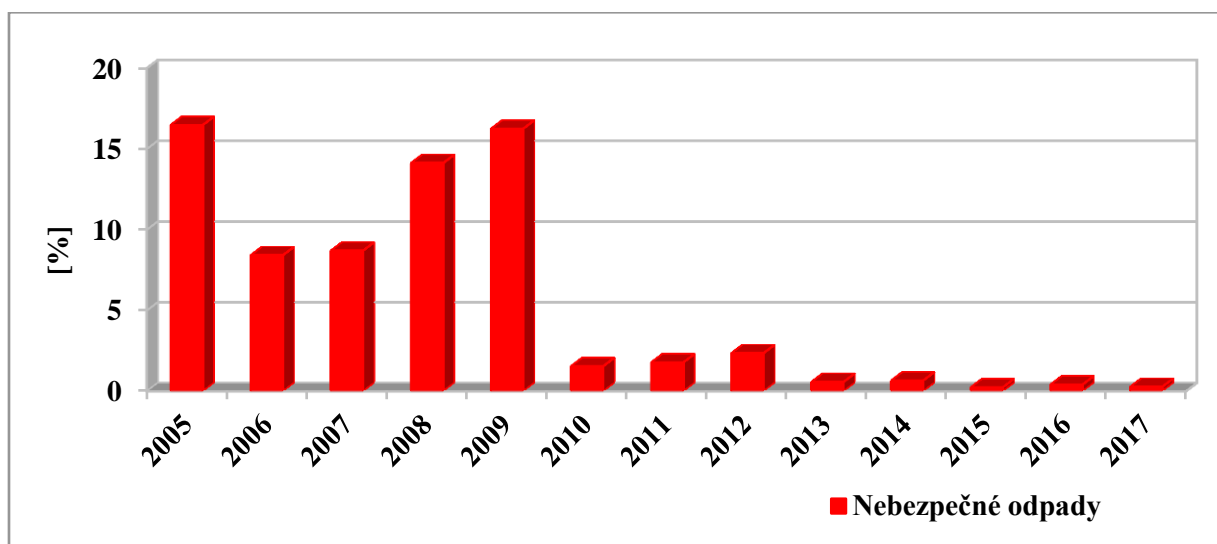
Graf č. 6: Podíl využitých nebezpečných odpadů v letech 2005 – 2017.
