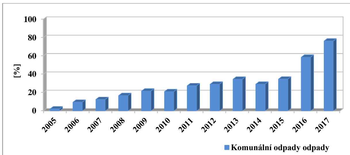
Graf č. 5: Podíl využitých komunálních odpadů v letech 2005 – 2017.
