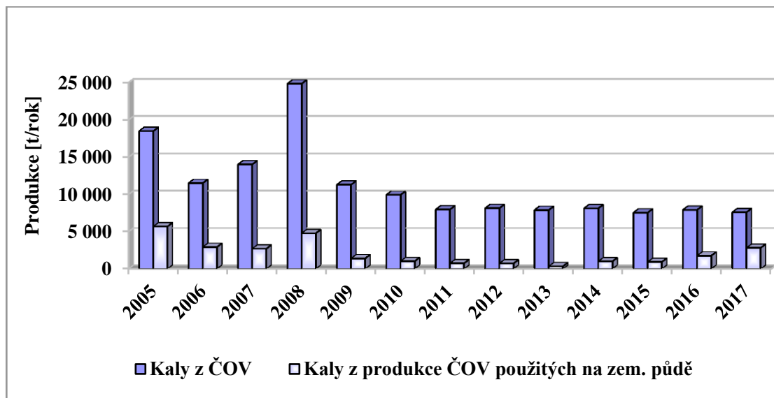
Graf č. 31: Srovnání produkce kalů z ČOV použitých na zemědělské půdě s celkovou produkcí kalů z ČOV v letech 2005 – 2017.
