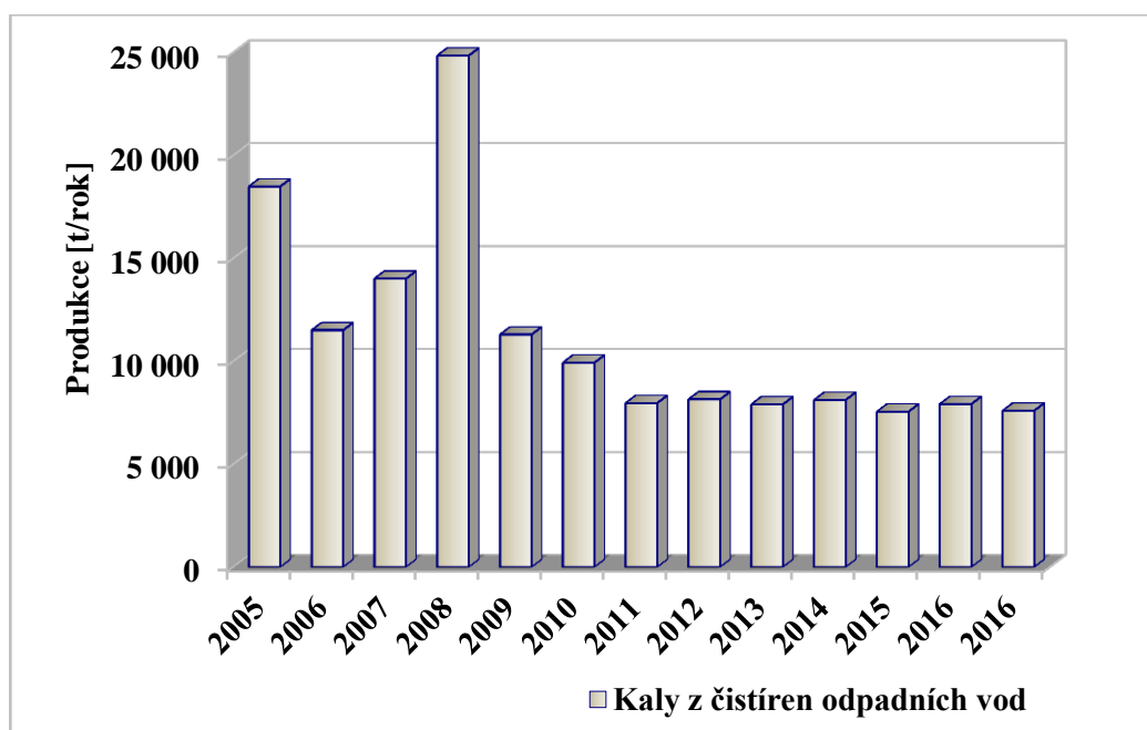
Graf č. 30: Celková produkce kalů z čistíren odpadních vod v letech 2005 – 2017.
