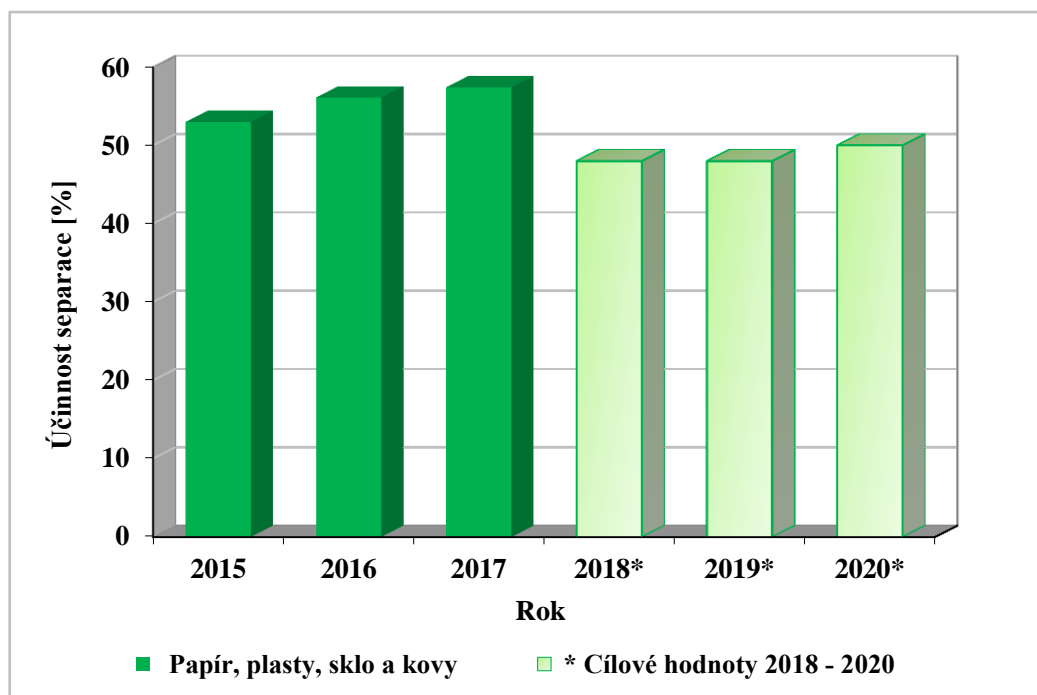
Graf č. 34. Účinnost tříděného sběru využitelných složek KO v období 2015 – 2017.
