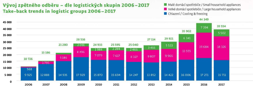
Graf č. 45: Vývoj zpětného odběru v letech 2006 – 2017 – ELEKTROWIN a.s.
