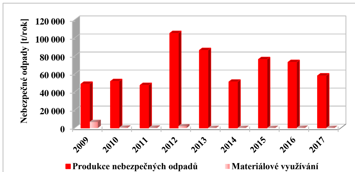
Graf č. 36: Produkce a materiálové využívání nebezpečných odpadů na území kraje.
