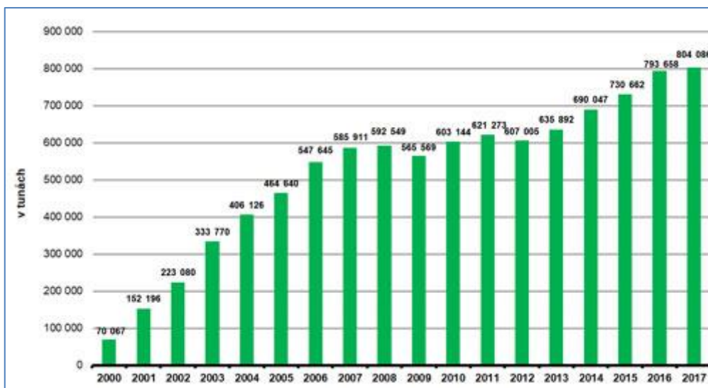
Graf č. 39: Celkové množství využitých odpadů z obalů.
