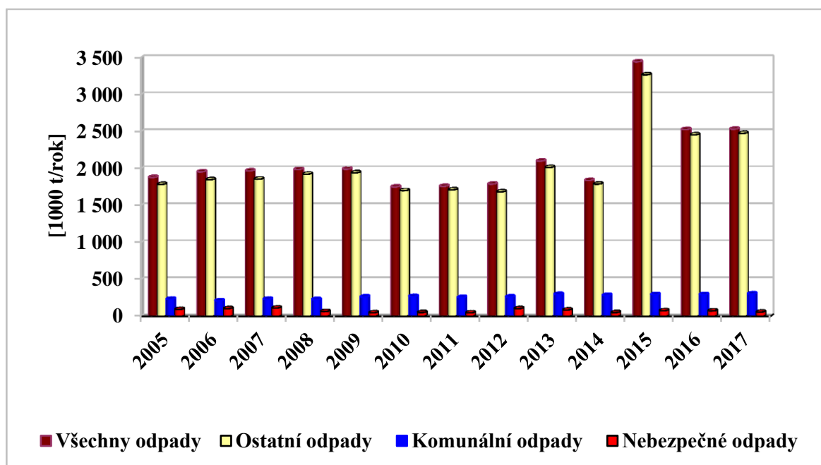
Graf č. 1: Celkové produkce odpadů v letech 2005 – 2017.
