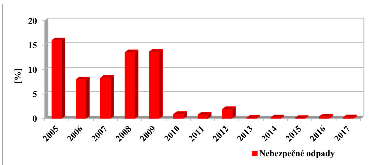
Graf č. 10: Podíl materiálově využitých nebezpečných odpadů v letech 2005 – 2017.
