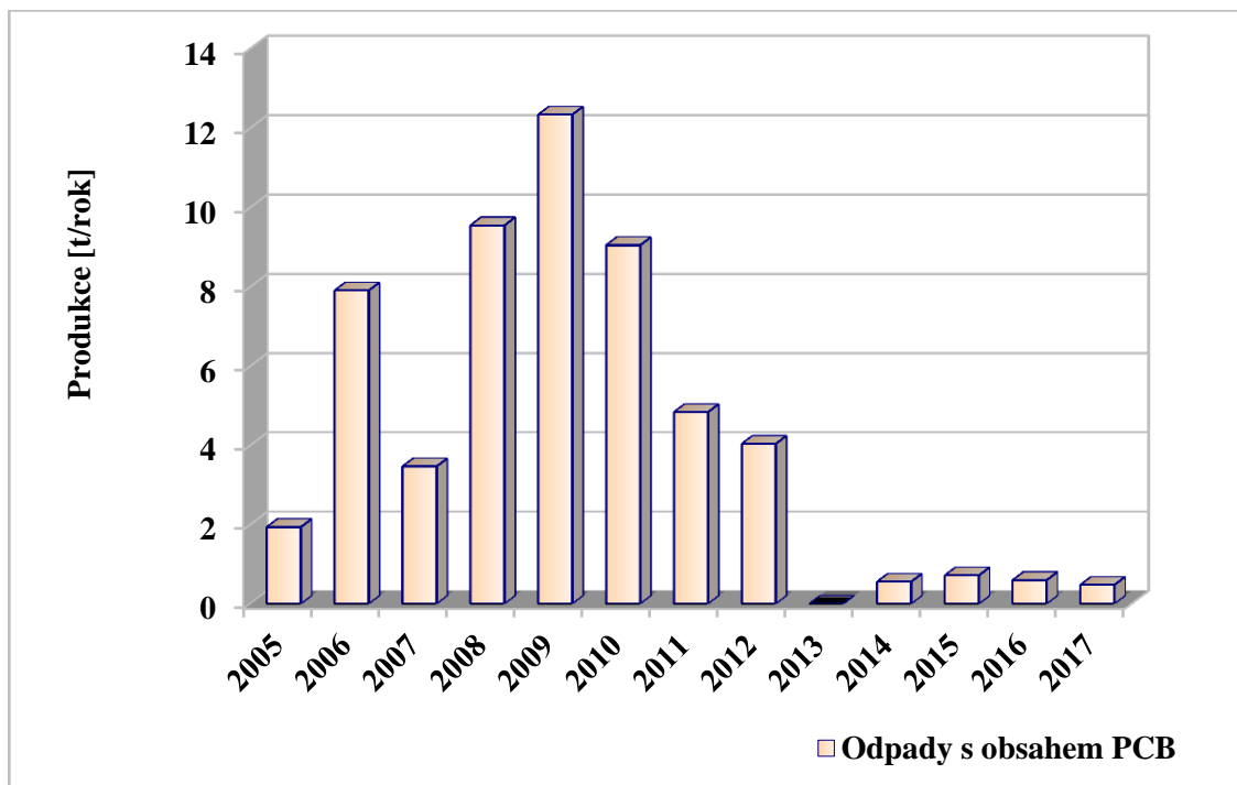
Graf č. 29: Celková produkce odpadů s obsahem PCB v letech 2005 – 2017.
