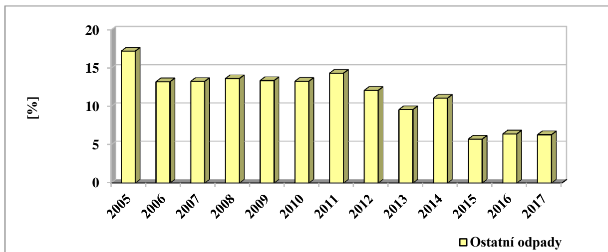
Graf č. 19: Podíl ostatních odpadů odstraněných skládkováním v letech 2005 – 2017.
