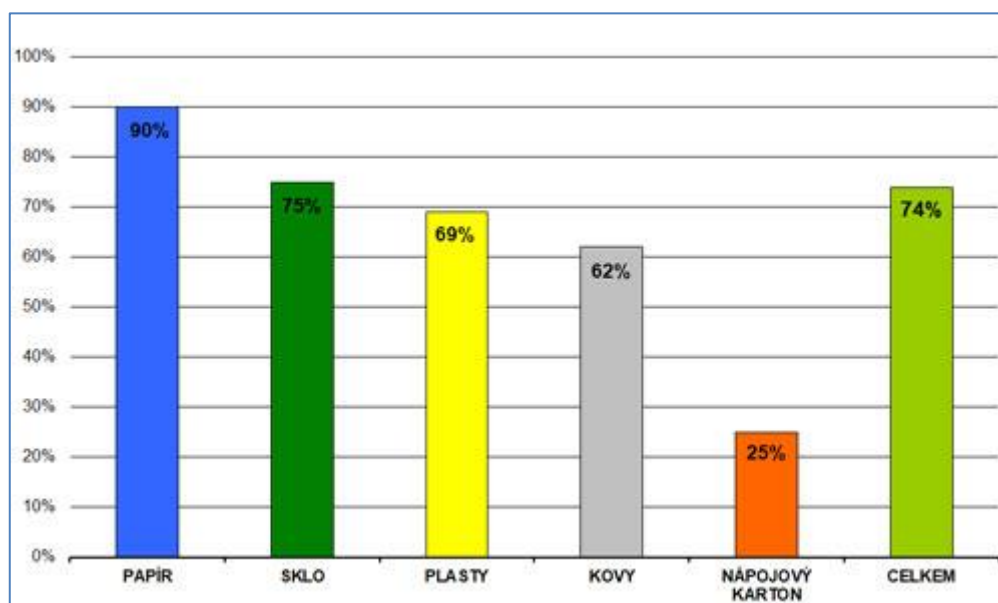
Graf č. 40: Dosažená míra recyklace a využití odpadů z obalů 2017.
