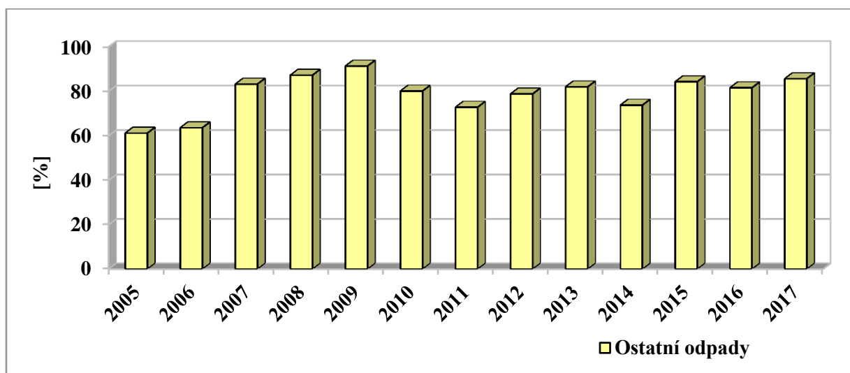
Graf č. 11: Podíl materiálově využitých ostatních odpadů letech 2005 – 2017.
