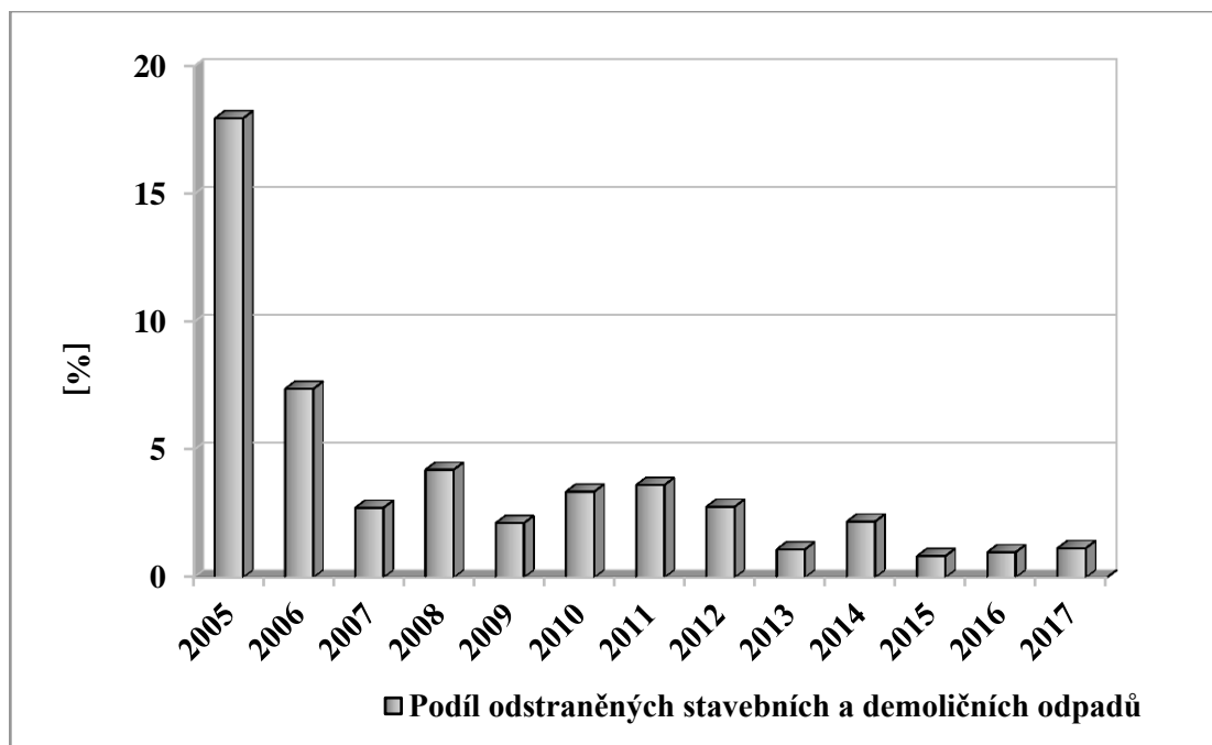
Graf č. 28: Podíl odstraněných stavebních a demoličních odpadů v letech 2005 – 2017.
