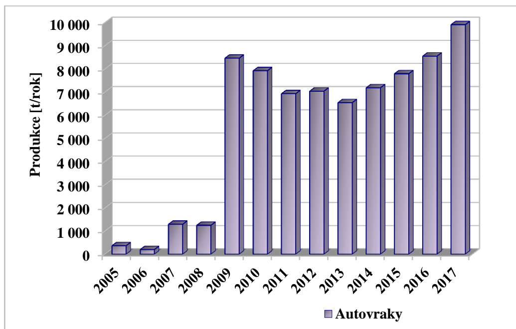
Graf č. 33: Celková produkce autovraků v letech 2005 – 2017.
