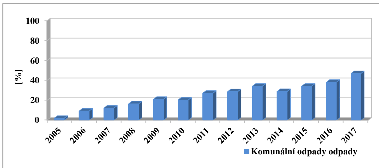
Graf č. 9: Podíl materiálově využitých komunálních odpadů v letech 2005 – 2017.
