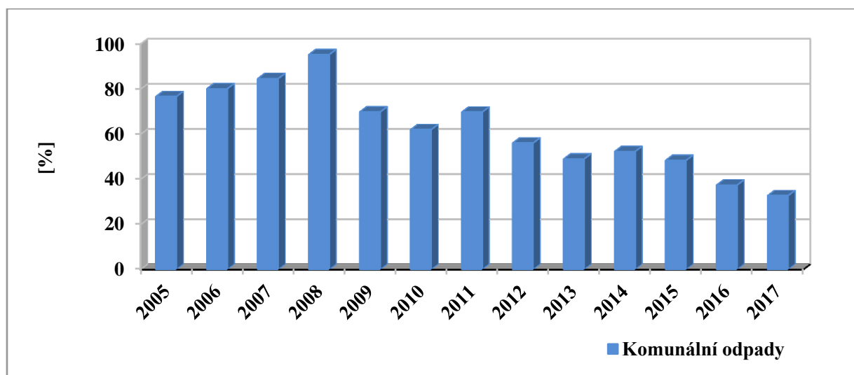
Graf č. 18: Podíl nebezpečných odpadů odstraněných skládkováním v letech 2005 – 2017.
