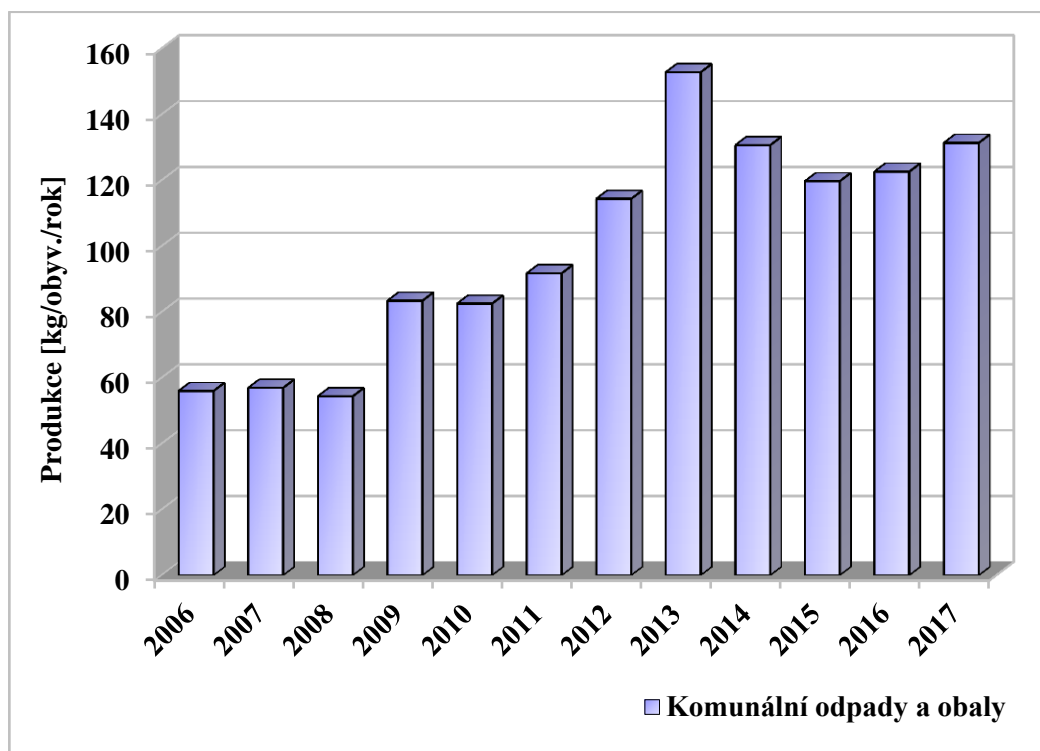
Graf č. 24: Produkce odděleného sběru komunálních odpadů a obalů na obyvatele v letech 2006 – 2017.
