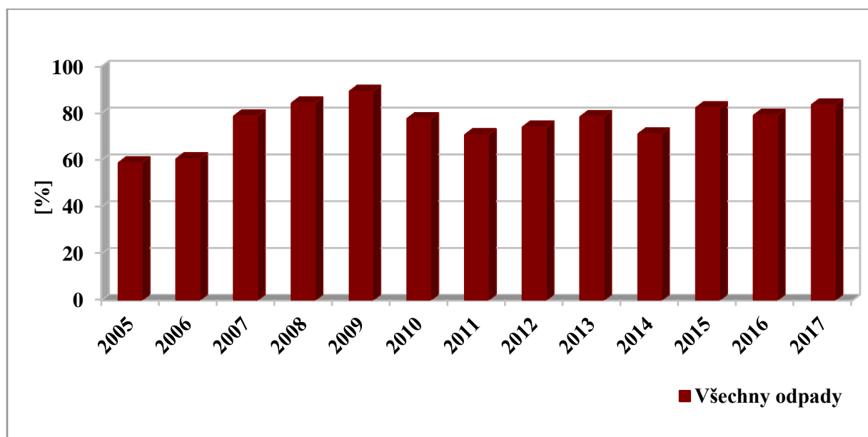
Graf č. 8: Podíl materiálově využitých všech odpadů v letech 2005 – 2017.
