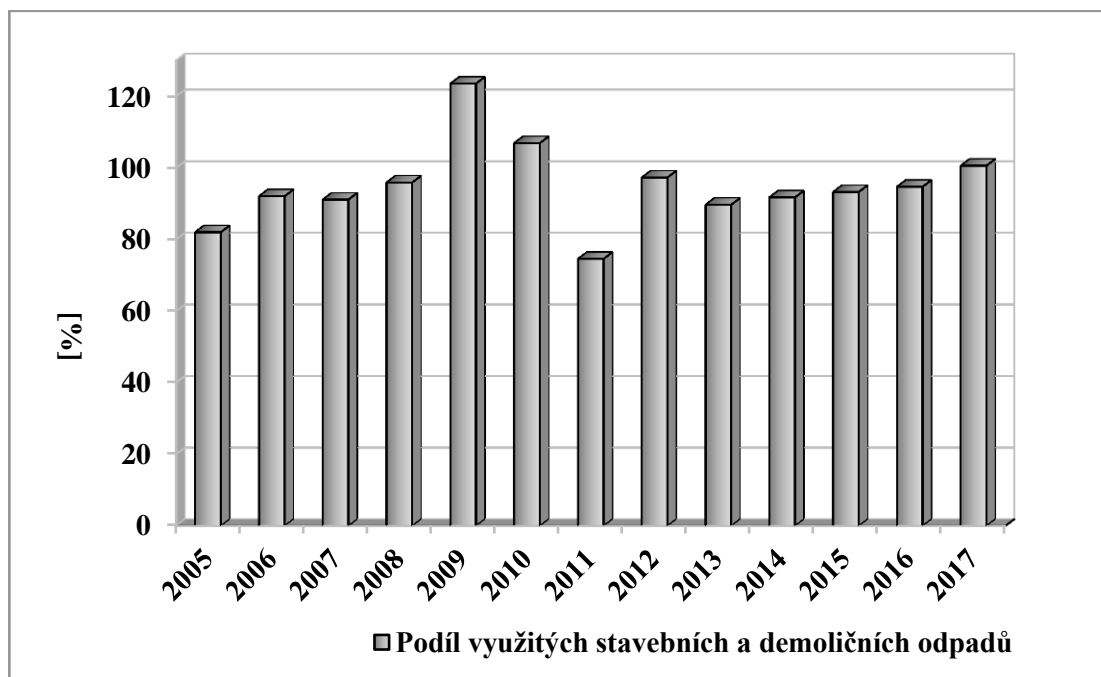
Graf č. 27: Podíl využitých stavebních a demoličních odpadů v letech 2005 – 2017
