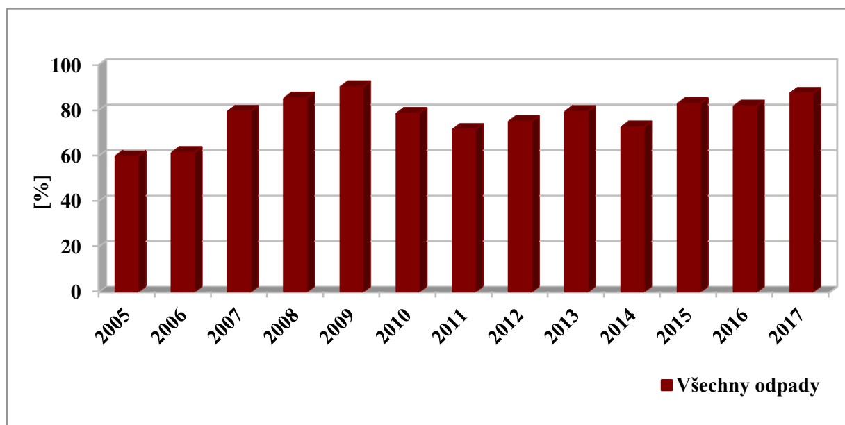
Graf č. 4: Podíl využitých všech odpadů v letech 2005 – 2017.
