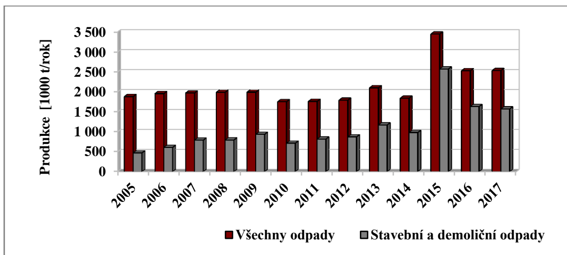
Graf č. 26: Srovnání produkce stavebních a demoličních odpadů s celkovou produkcí odpadů v letech 2005 – 2017.
