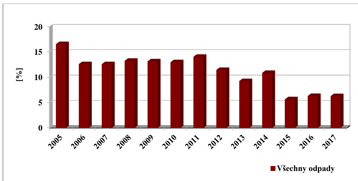
Graf č. 16: Podíl všech odpadů odstraněných skládkováním v letech 2005 – 2017.
