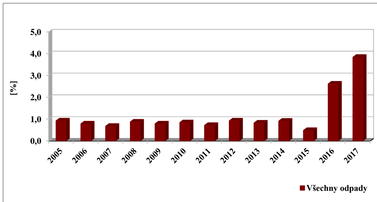
Graf č. 12: Podíl všech energeticky využitých odpadů v letech 2005 – 2017.
