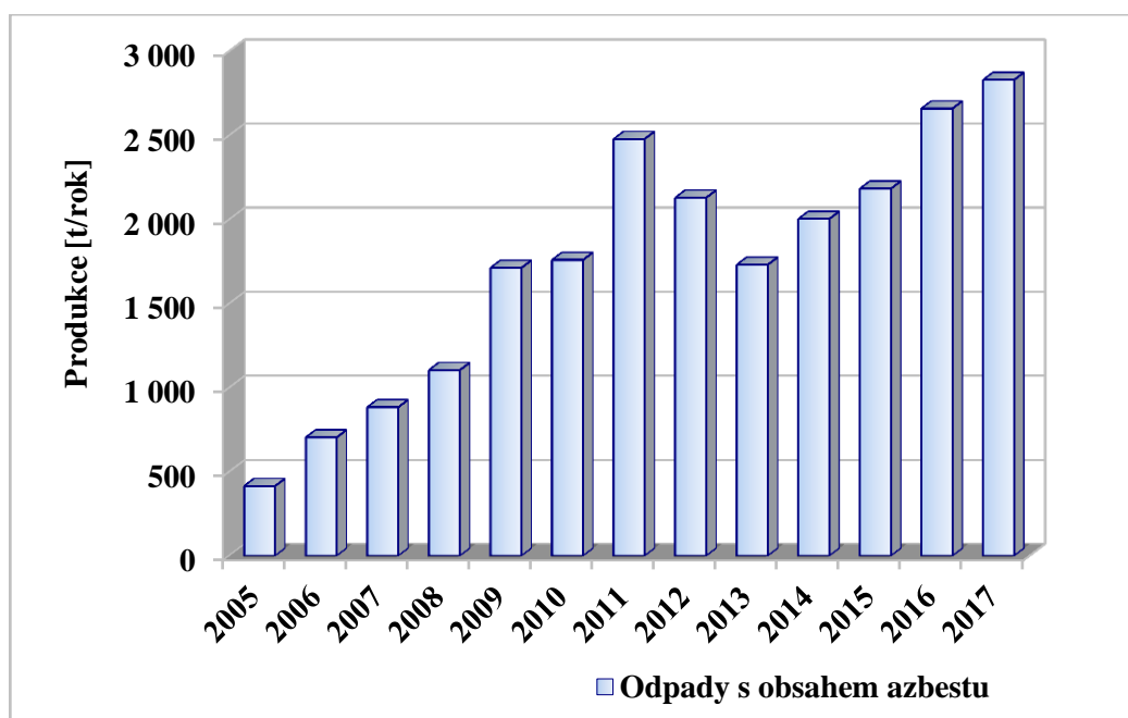
Graf č. 32: Celková produkce odpadů s obsahem azbestu v letech 2005 – 2017.
