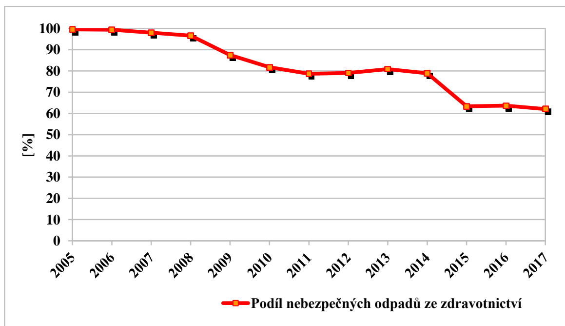
Graf č. 23: Podíl nebezpečných odpadů ze zdravotnictví na celkové produkci odpadů ze zdravotnictví v letech 2005 – 2017.
