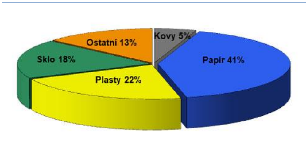
Graf č. 38: Struktura nevratných obalů 2017.
