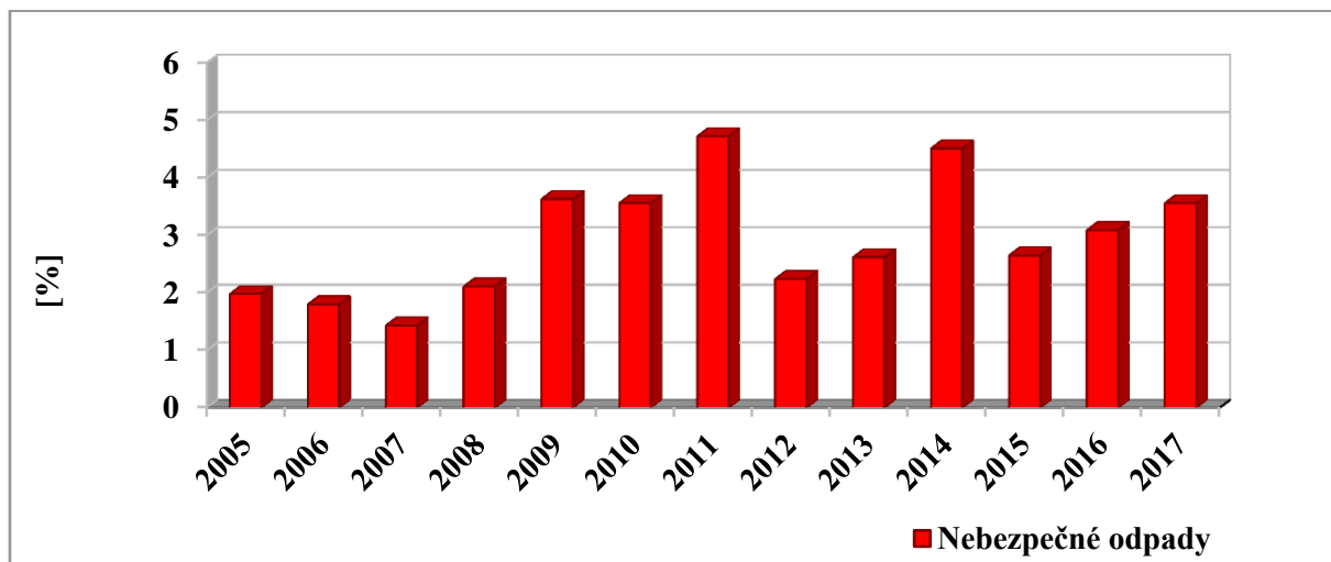
Graf č. 21: Podíl nebezpečných odpadů odstraněných spalováním v letech 2005 – 2017.
