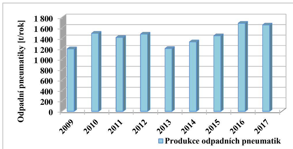
Graf č. 48: Produkce odpadních pneumatik na území kraje.
